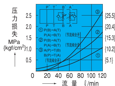
OCY-G03-W-Y-J51 (OCY-G03-W-X-J51)
