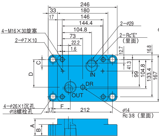
MES-06*-10
