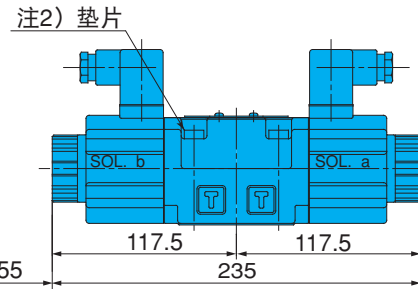
线圈装卸尺寸
