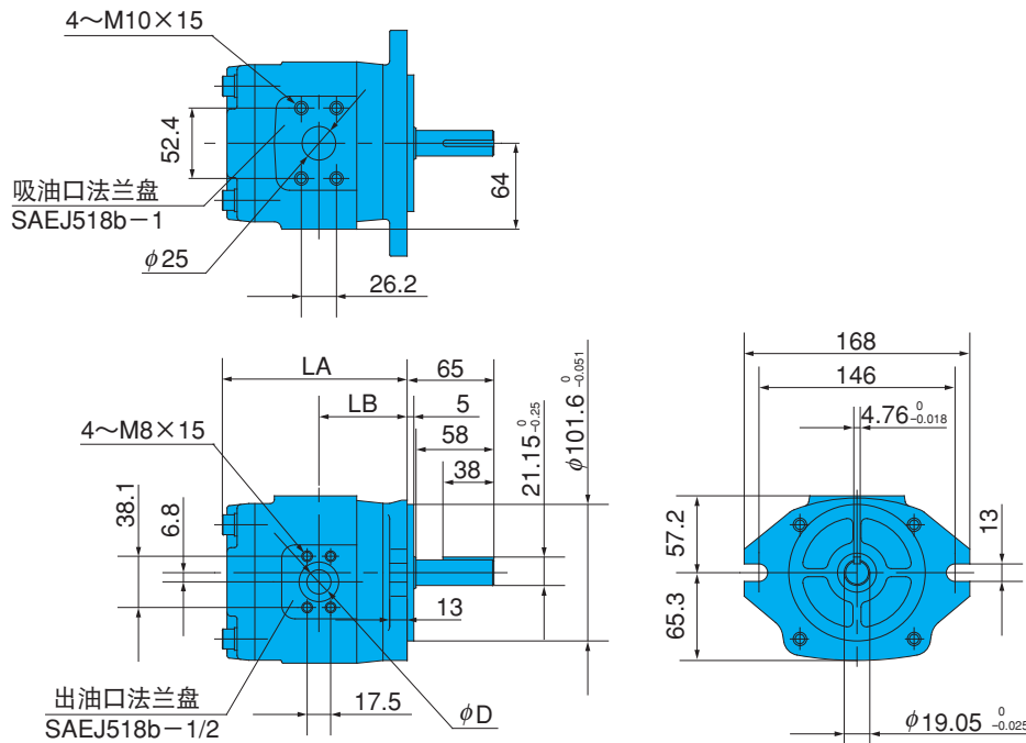
IPH-3B-*-20 (法兰式右转)
