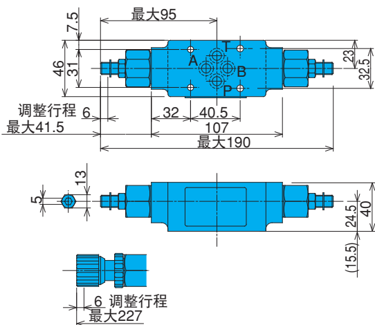
OCY-G01-W-X-Y-20
