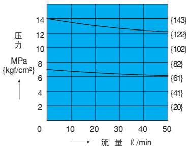
OG-G01-P 2 -21
