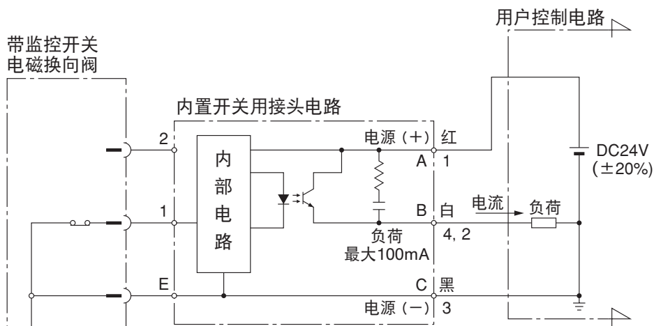
与带开关接头的连接方法
