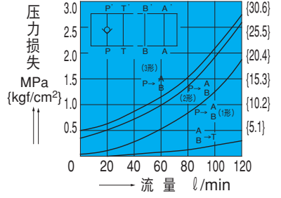
OC-G03-P*-J50
