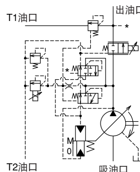
PZ-6B
