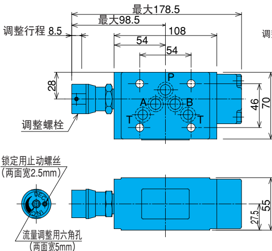
OF-G03-P60-J50
