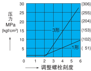
OR-G01-P*-20
