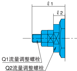
流量调节长度和泵排量
