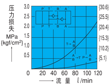
OCV-G03-W-J50
