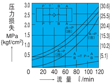
OC-G03-AP*-J50
