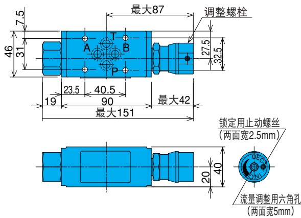
OF-G01-P20-20
