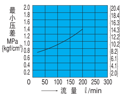
OFH-G04-W200-Y-10
