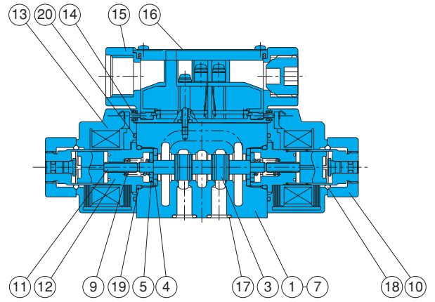
SL-G01-C ** -R-C *-31
