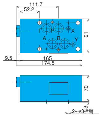
OCH-G04-T*-10
