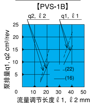
流量调节长度和泵排量
