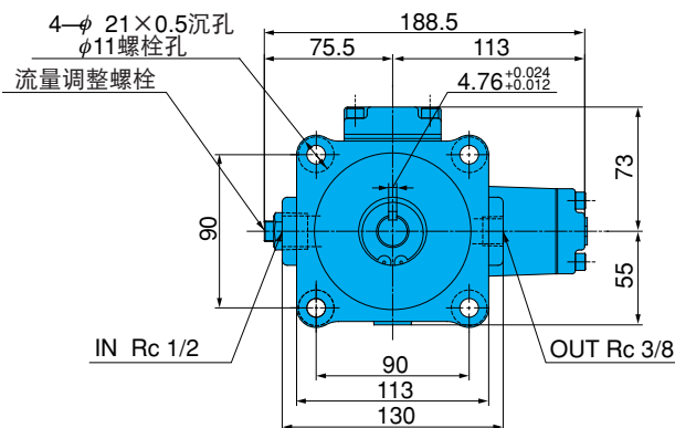
VDR-1B-*-13（法兰式）
