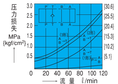
OC-G03-T*-J50
