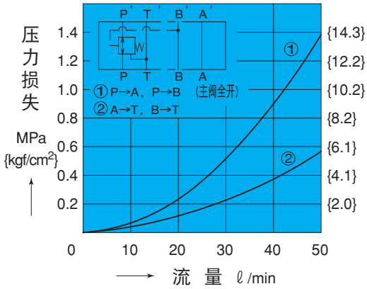
OG-G01-B*-21
