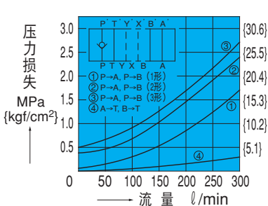
OCH-G04-P*-10
