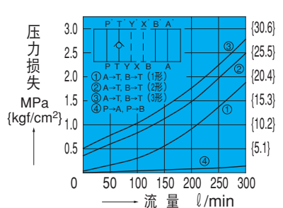
OCH-G04-T*-10
