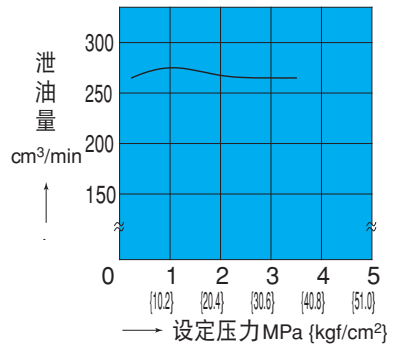
OG-G03-BC-J51
