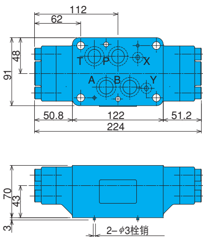
OPH-G04-**- (D)-10
