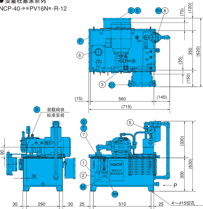
P箭头指示图
