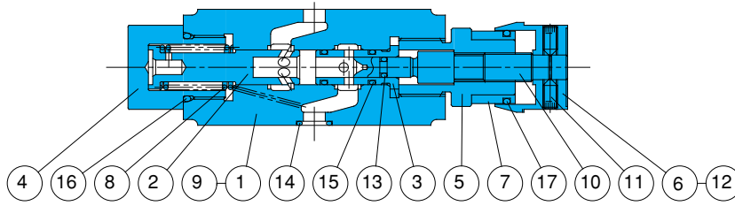
密封部件一览表 (组件型号 BFBS-01FP)
