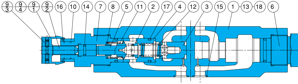
密封部件一览表 (组件型号 BFES-03CF*)
