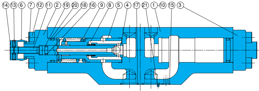
密封部件一览表 (组件型号 BFKS-04CF*)
