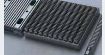
ステアリングラックのプローチ加工
