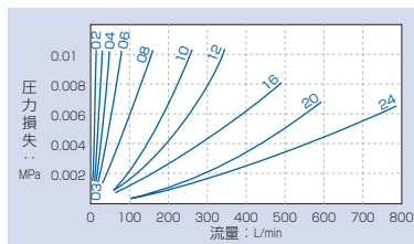
ろ過精度150メッシュ (150K)
