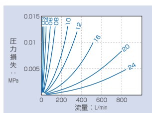
ろ過精度60メッシュ (60W)
