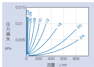
ろ過精度150メッシュ (150W)
