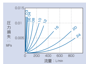
ろ過精度100メッシュ (100W)
