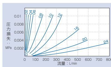
ろ過精度100メッシュ (100K)
