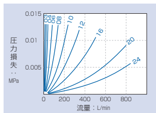
ろ過精度150メッシュ (150W)
