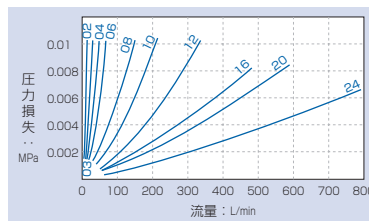
ろ過精度200メッシュ (200K)
