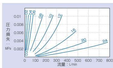
ろ過精度60メッシュ (60K)
