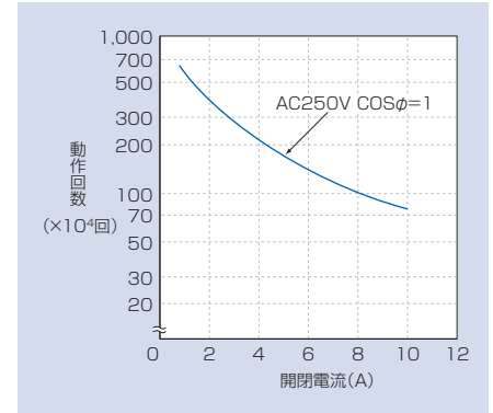
電気的寿命曲線
