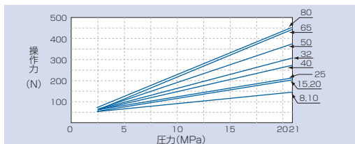
(弁閉止ハンドル操作力線図)
