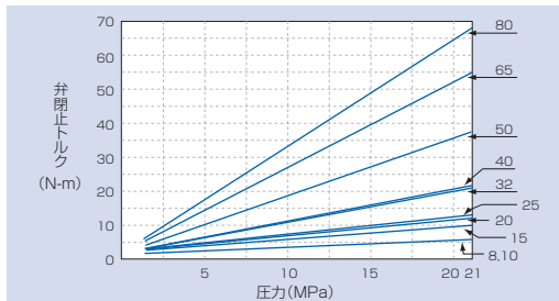
(弁閉止ハンドル操作力線図)
