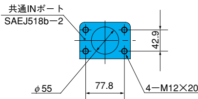
A矢視
