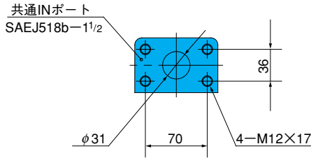
A矢視
