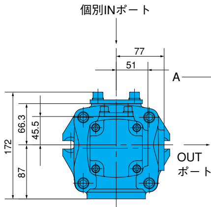
A矢視
