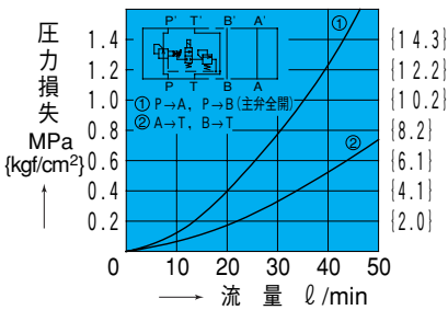
圧力-流量特性 OGS-G01-P21-K-**-22 (2形)
