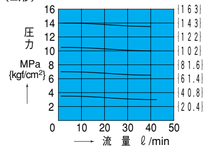
圧力-流量特性 OGS-G01-P21-K-**-22 (2形)
