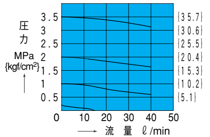
OGS-G01-P*C-K-**-22 (C形)
