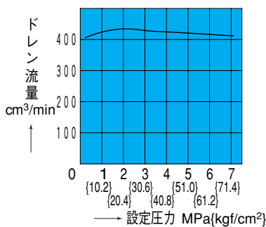
圧カードレン流量特性 OGS-G01-PIC-K-**-22
