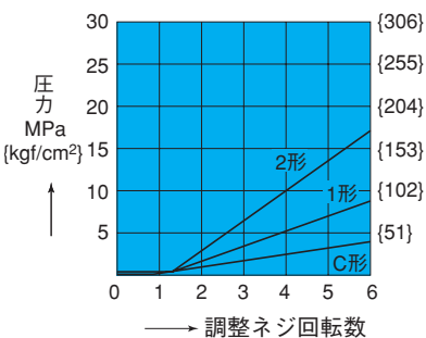
調整ネジ回転数-圧力特性 OGS-G01-P**-22
