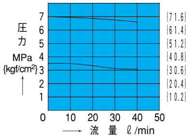
圧力-流量特性 OGS-G01-PIC-K-**-22 (1形)
