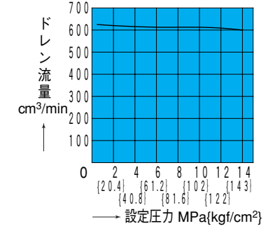
圧カードレン流量特性 OGS-G01-P21-K-**-22
