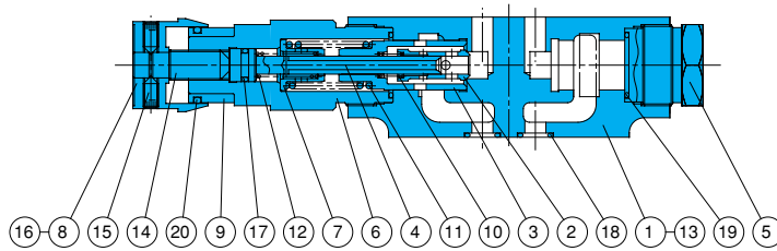
シール部品一覧表 (キット形式 BFCS-01CF*)
