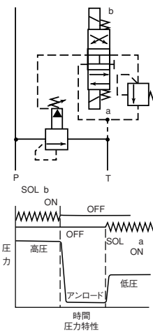
(二圧制御回路例)
